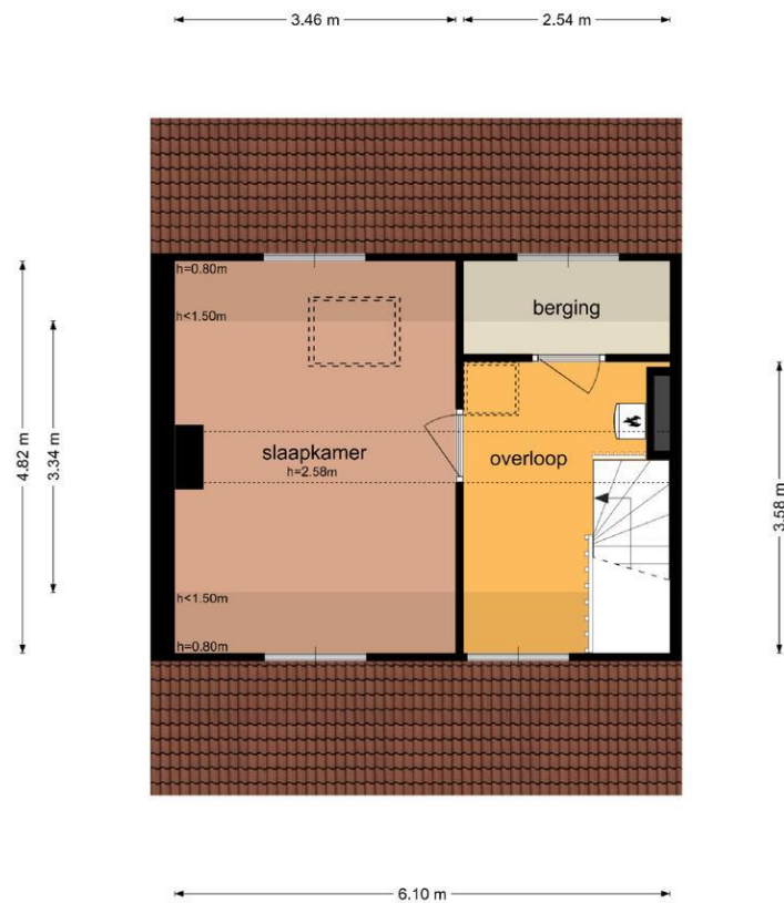
Rijksstraatweg 148 - Loenen aan de Vecht Tweede Verdieping
